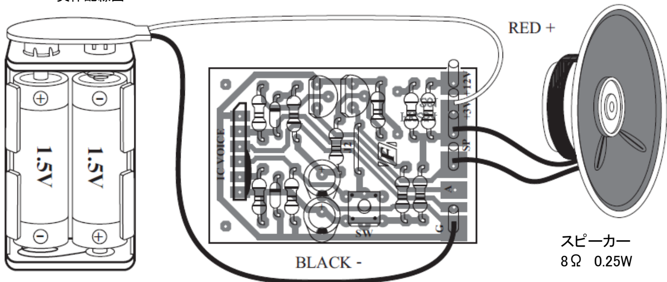
実体配線図
