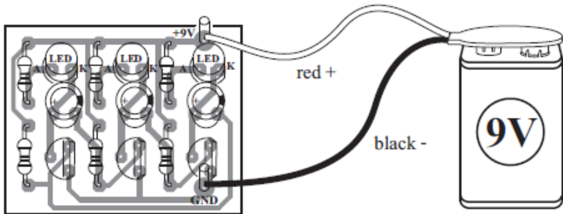
実体配線図
