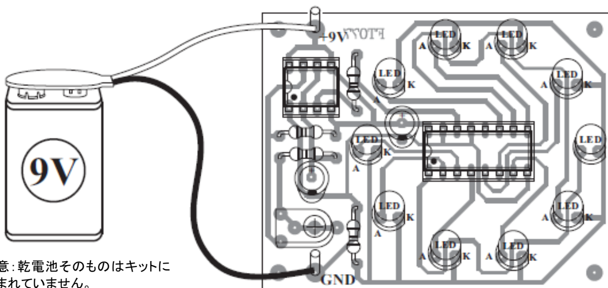
実体配線図
