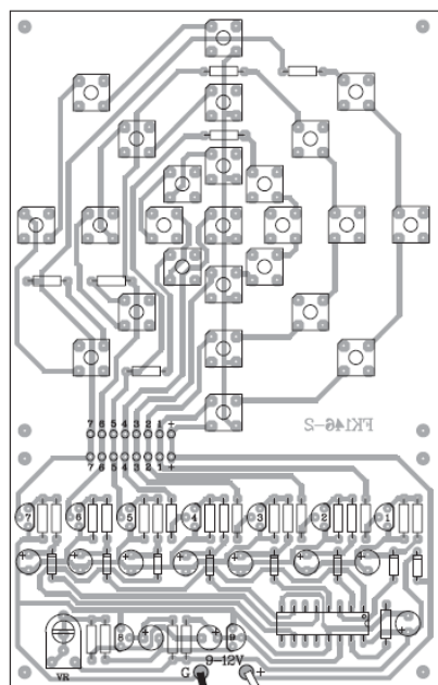
実体配線図
