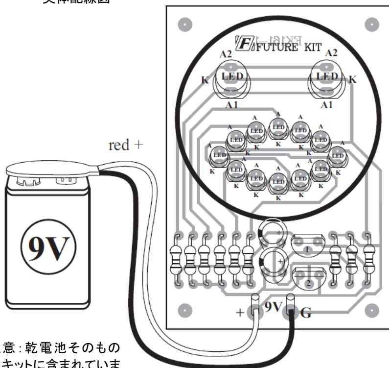
実体配線図
