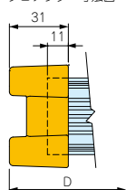
AWPシリーズ プロテクター寸法図
