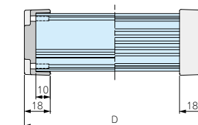
AWPシリーズ プロテクター寸法図
