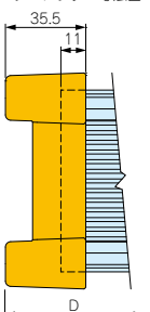
AWPシリーズ プロテクター寸法図
