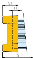
AWPシリーズ プロテクター寸法図
