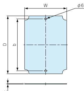
BMP0912Z～1727Z外観寸法図
