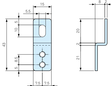
CK-35P外観寸法図
