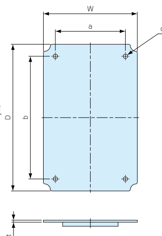
BMP1928P～4050P(リブ付) 外観寸法図
