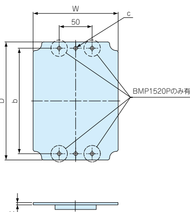
BMP1520P, 1525P(リブ付) 外観寸法図
