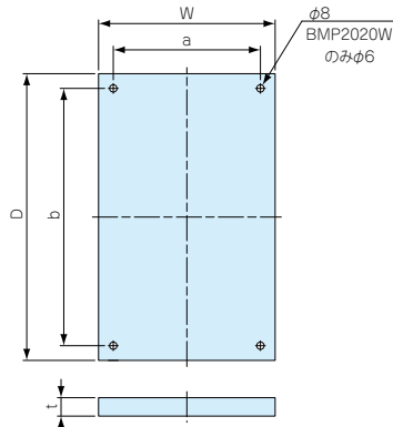
BMP1928W～4060W外観寸法図
