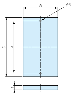
BMP0912W～1727W外観寸法図
