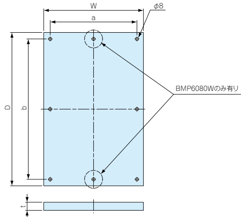
BMP5060W～6080W外観寸法図
