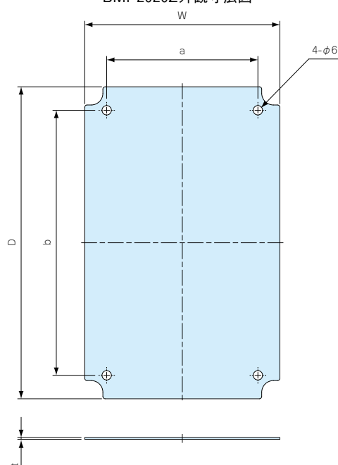
BMP2020Z外観寸法図
