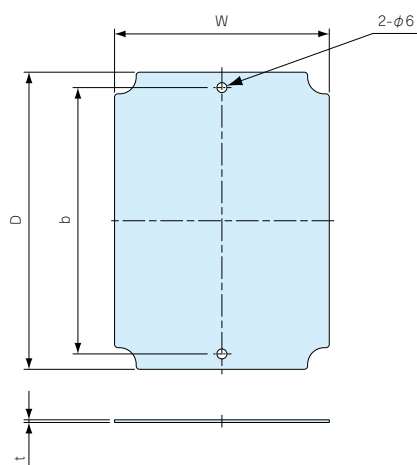
BMP0506Z～1525Z外観寸法図
