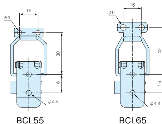
ラッチ寸法図
