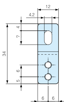
CK-34Z外観寸法図
