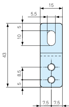
CK-35P外観寸法図
