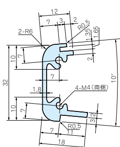
CF□-18フロントフレーム
