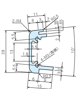
CF□-11フロントフレーム
