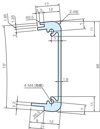
CF□-18リヤフレーム
