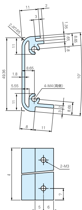
CF□-28フロントフレーム
