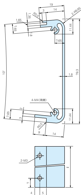
CF□-23リヤフレーム
