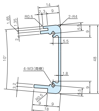
CF□-11リヤフレーム
