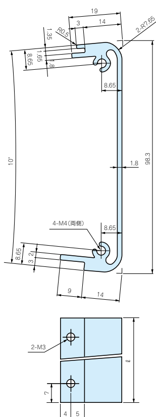
CF□-28リヤフレーム
