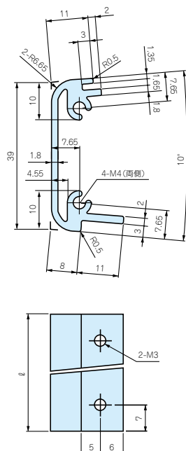
CF□-23フロントフレーム
