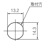
取付穴寸法図
