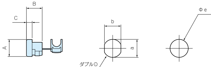
推奨取付穴寸法図 簡易取付穴寸法図
