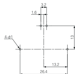
推奨基板加工寸法
