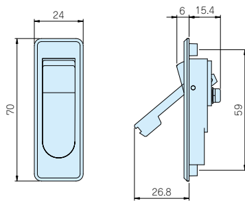
鍵無タイプ
