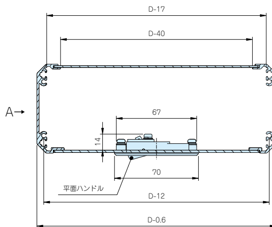
D方向図
