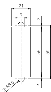
パネルカット寸法
