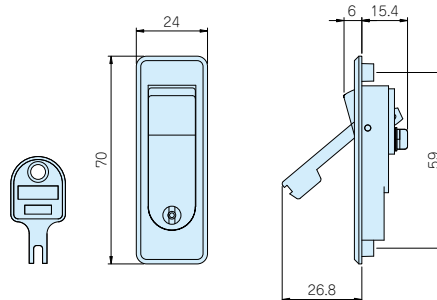
鍵付タイプ
