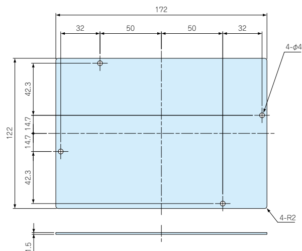
HQP26-18・HQP27-17外観寸法図
