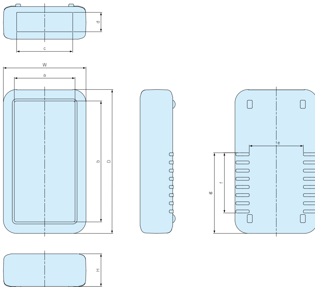
LCS135/LCS135H外観寸法図
