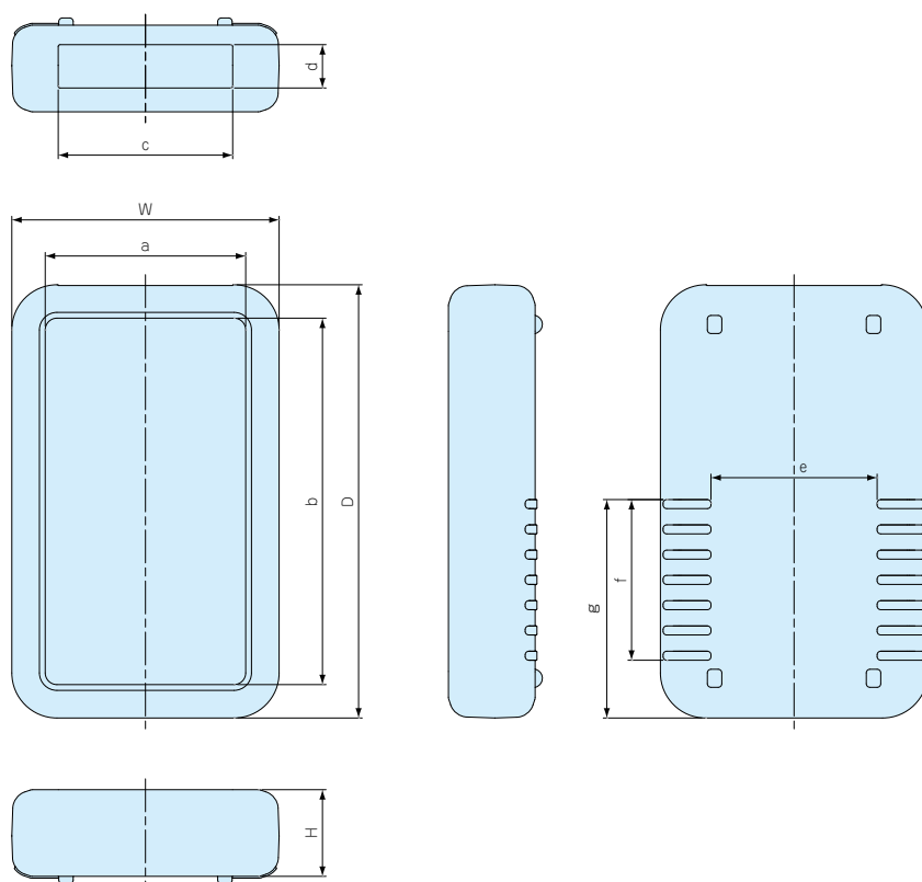
LCS115/LCS115H外観寸法図
