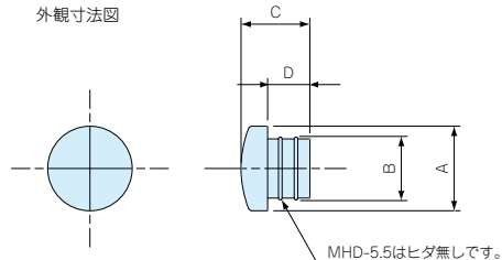
外観寸法図
