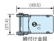
締付け金具
