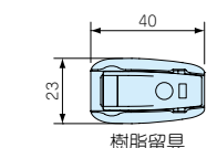
樹脂留具
