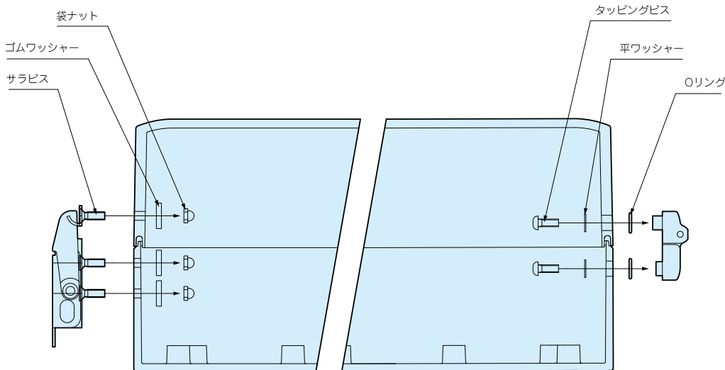
ラッチ、ヒンジ取付け方法
