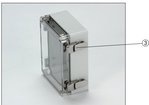
ラッチ、ヒンジ取付け方法
