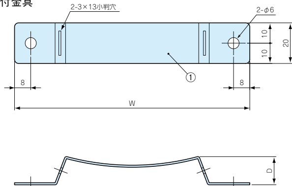
取付金具
