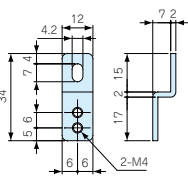
CK-34Z
