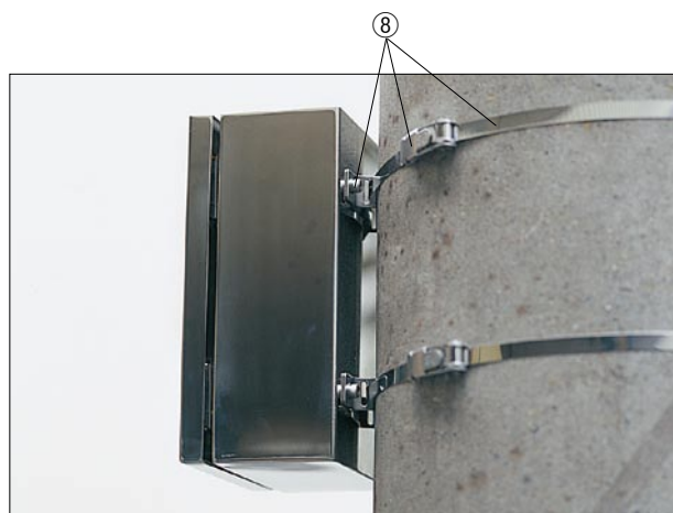
取付金具
