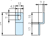
CK-34N
