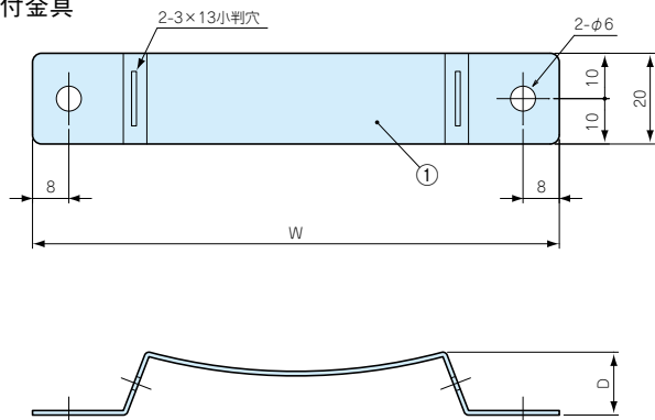
取付金具
