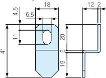
CK-26N
