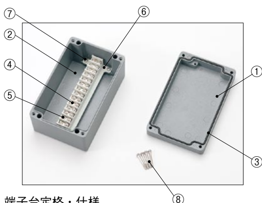
端子台定格・仕様
