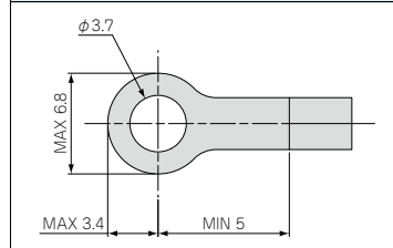
適合圧着端子 R1.25-3.5
